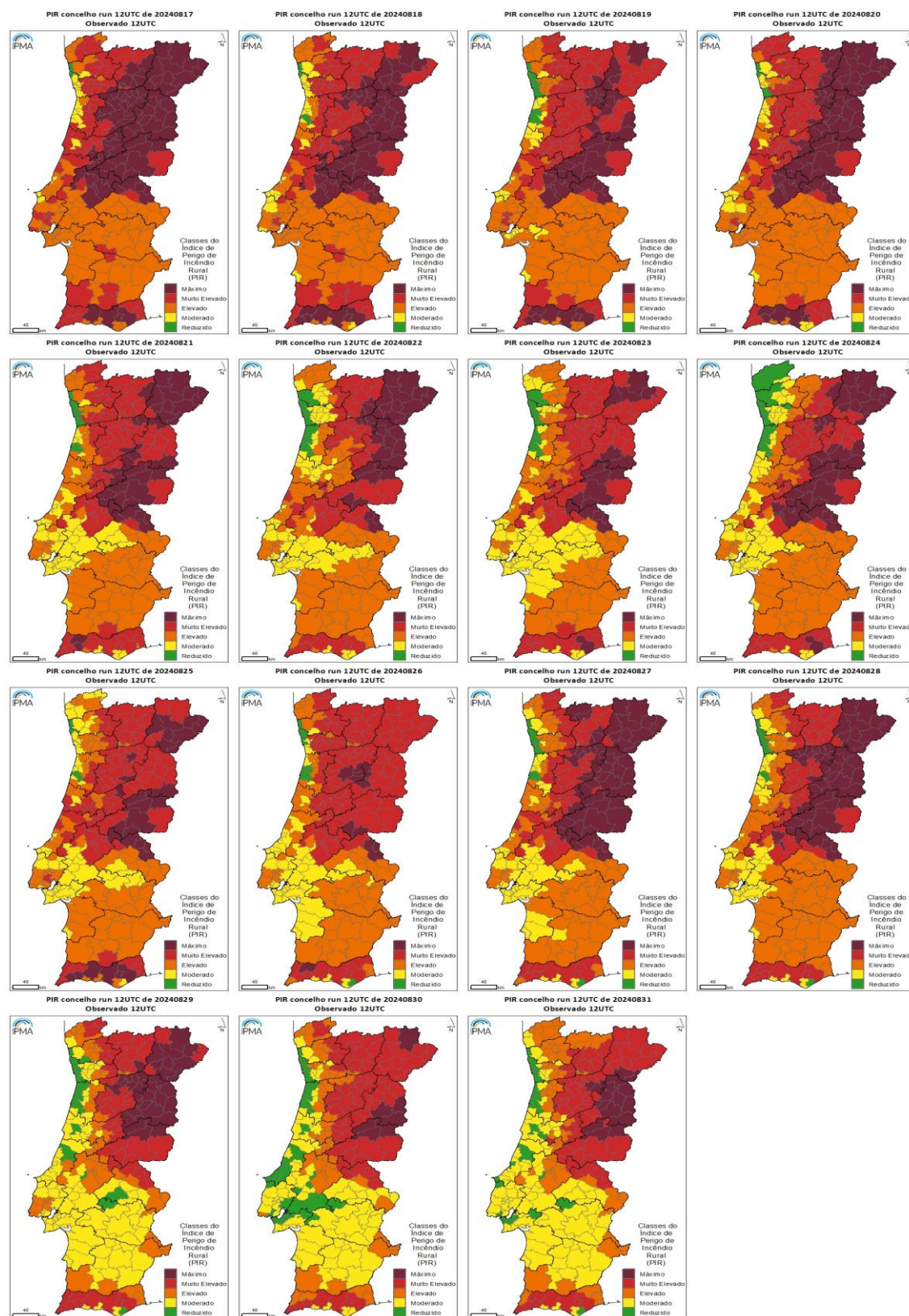
Figura AIII.2 – Mapas das classes do PIR observado a nível de Concelho, agosto de 2024 (dias 17 a 31).
