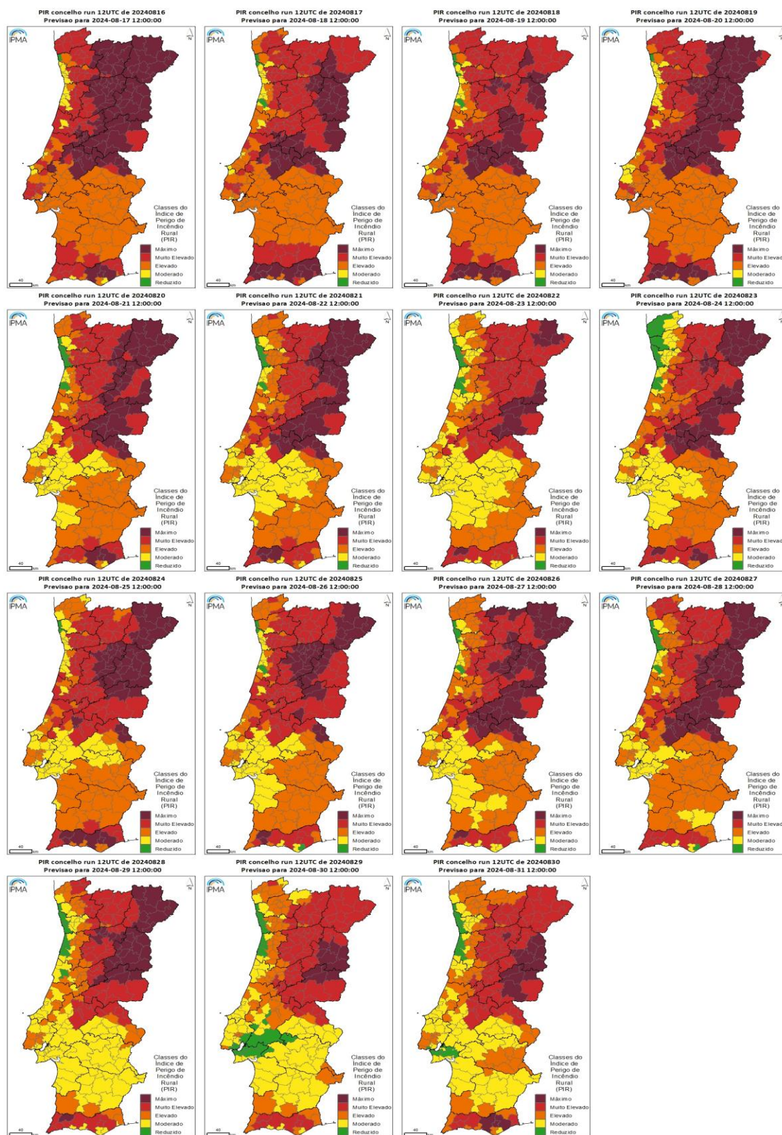
Figura AIII.4 – Mapas das classes do PIR, previsão a nível de Concelho, agosto de 2024 (17 a 31).
