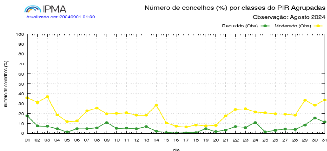
Figura 9 - Evolução diária em agosto da percentagem de concelhos nas classes de PIR. (a) Elevado Muito Elevado ou Máximo (laranja), Muito Elevado ou Máximo (vermelho), (b) Reduzido (verde), Moderado (amarelo).
