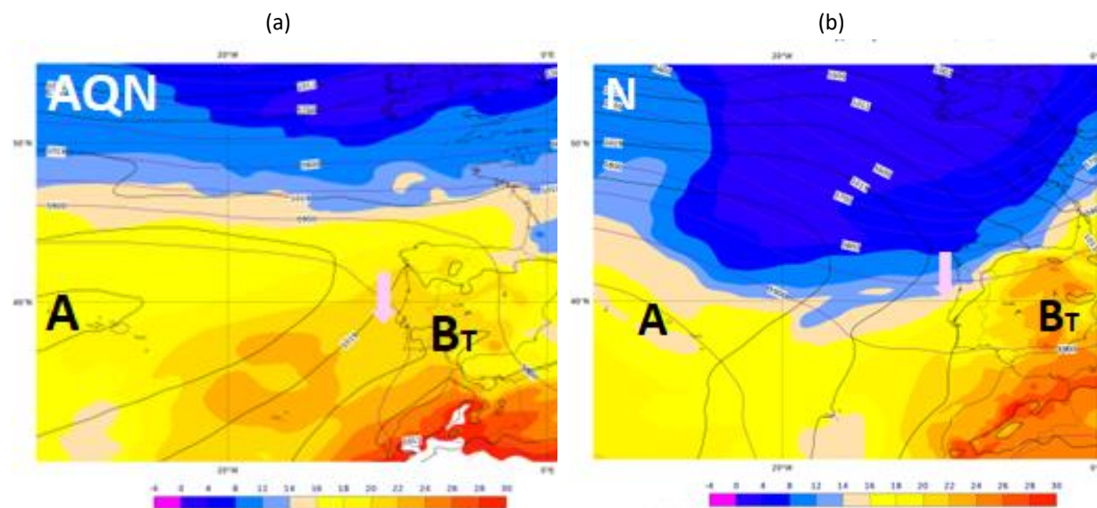
Figura 2 - Tipos de Tempo agosto de 2024: ECMWF(ERA5) às 12 UTC. Pressão ao nível médio do mar (linhas a preto, 4 em 4 hPa hPa), altura do geopotencial aos 500 hPa (linhas violeta a tracejado, 50 em 50 m), temperatura aos 850 hPa (cor, °C). (a) WTAQN (anticiclónico e fluxo quadrante norte, 16 agosto), (b) WTN (fluxo de norte, 24 agosto). A- Anticiclone, B- Depressão, B T - Depressão Térmica, seta a violeta - direção do fluxo.
