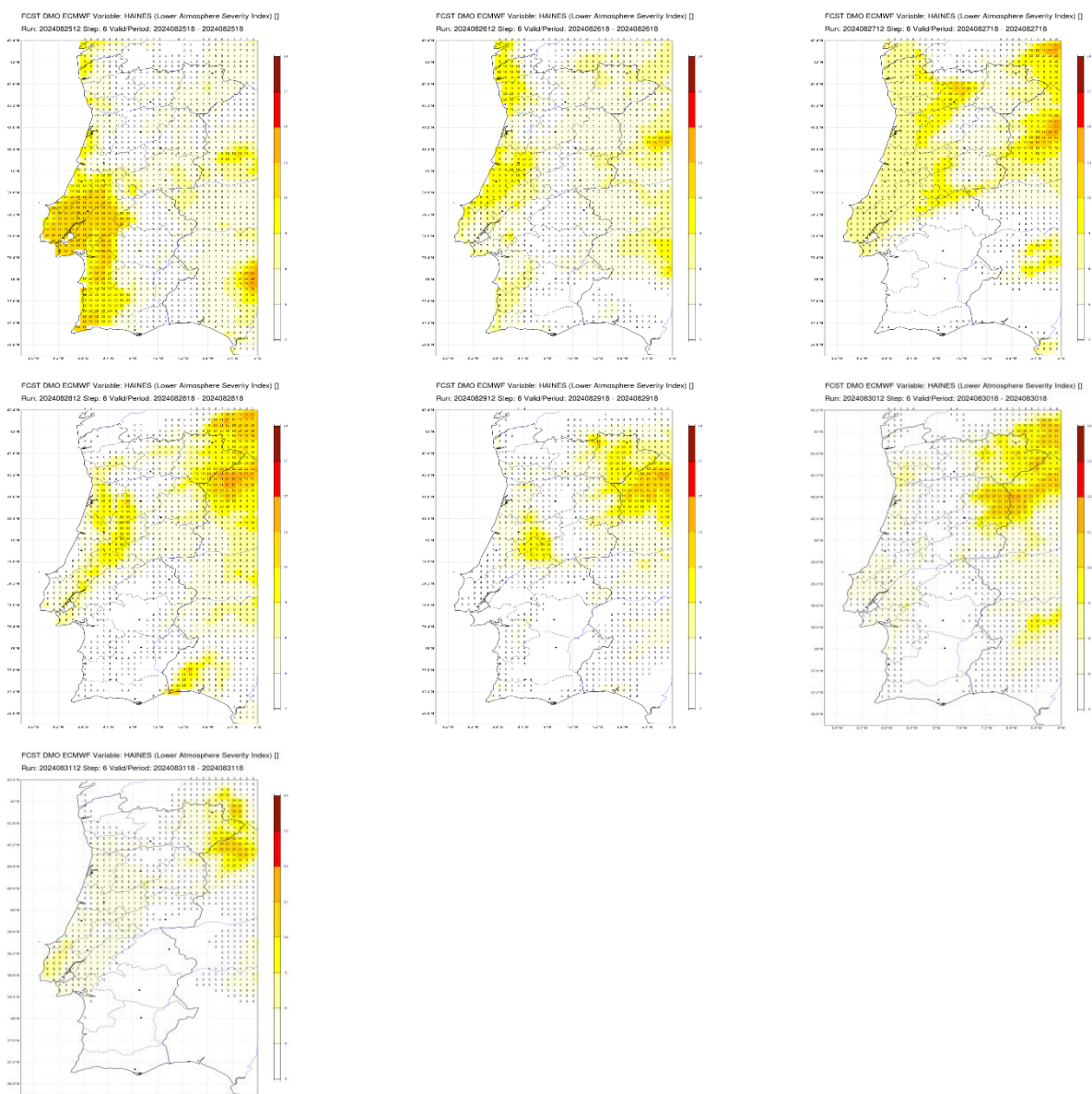
Figura AV.3 – Mapas do índice Haines, dias 25 a 31 agosto de 2024. Dias com trovoadas: 29 e 30
