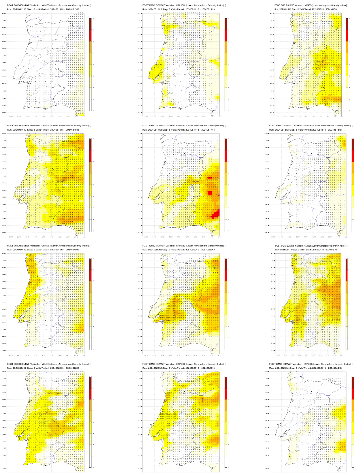
Figura AV.2 – Mapas do índice Haines, dias 13 a 24 agosto de 2024.
