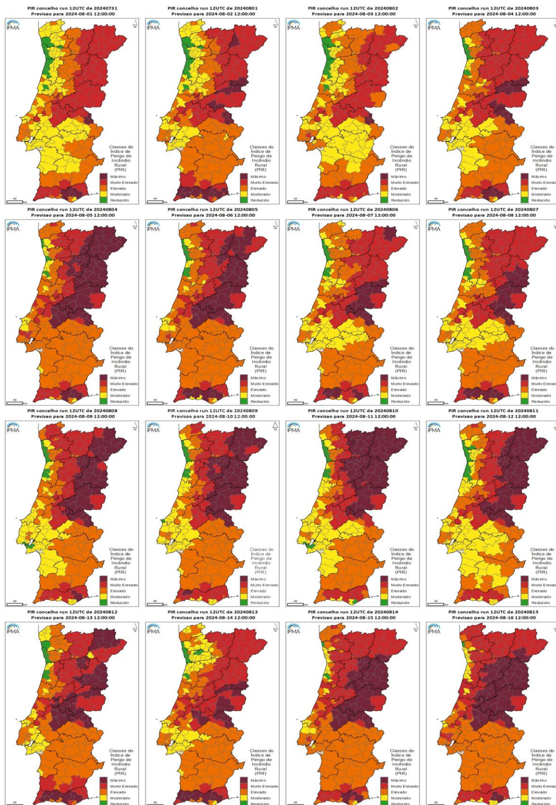
Figura AIII.3 – Mapas das classes do PIR, previsão a nível de Concelho, agosto de 2024 (dias 1 a 16).
