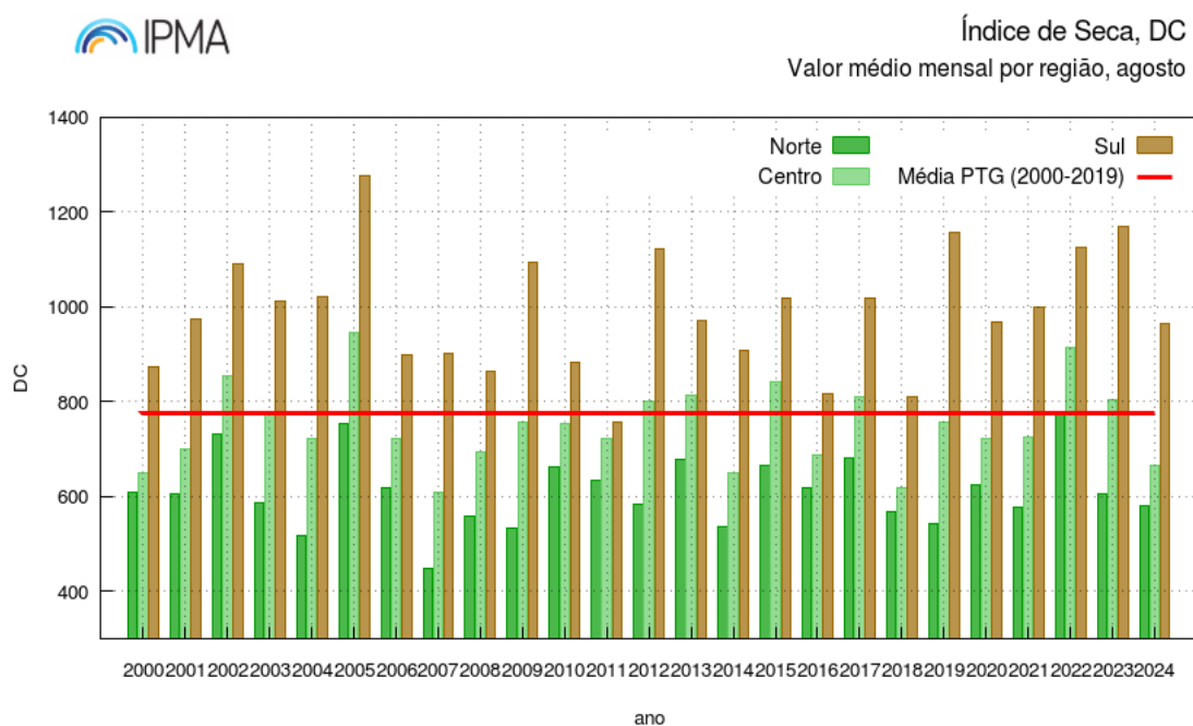
Figura 5 - Valor médio dos índices de seca, DC.
