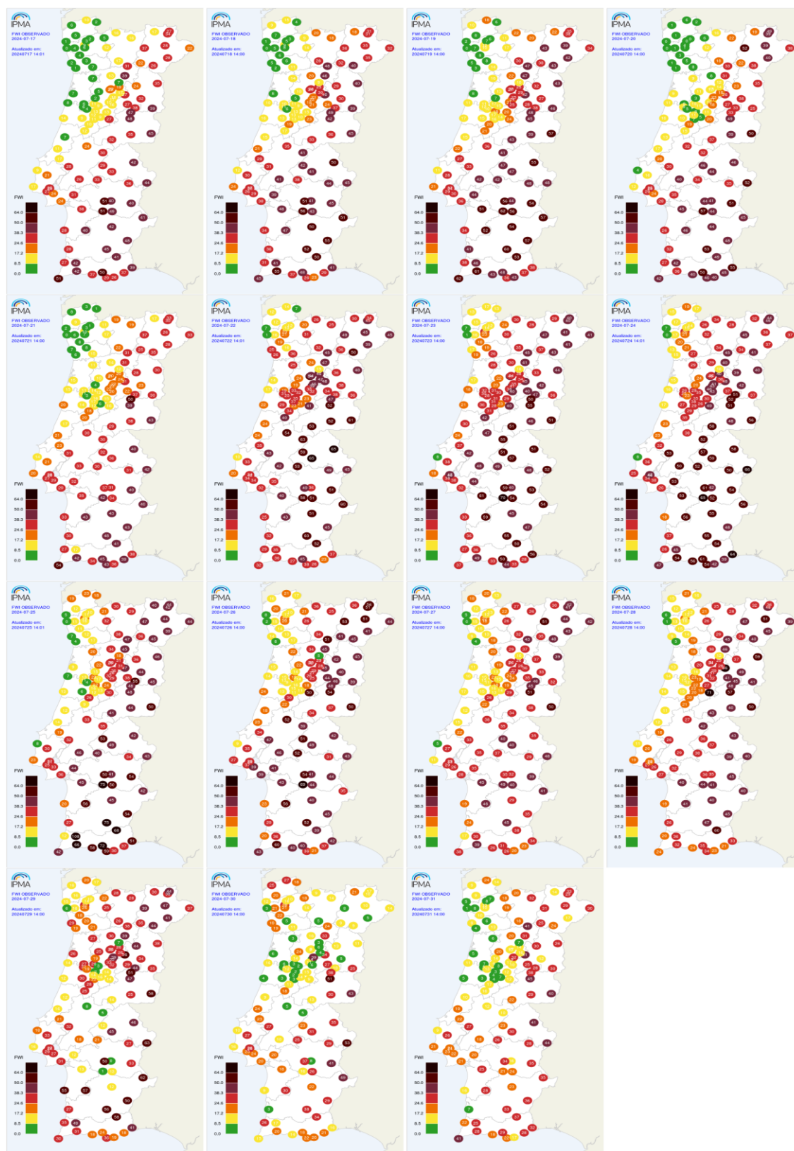
Figura AII.2 – Mapas do FWI Observado nas estações meteorológicas, agosto de 2024 (dias 17 a 31).
