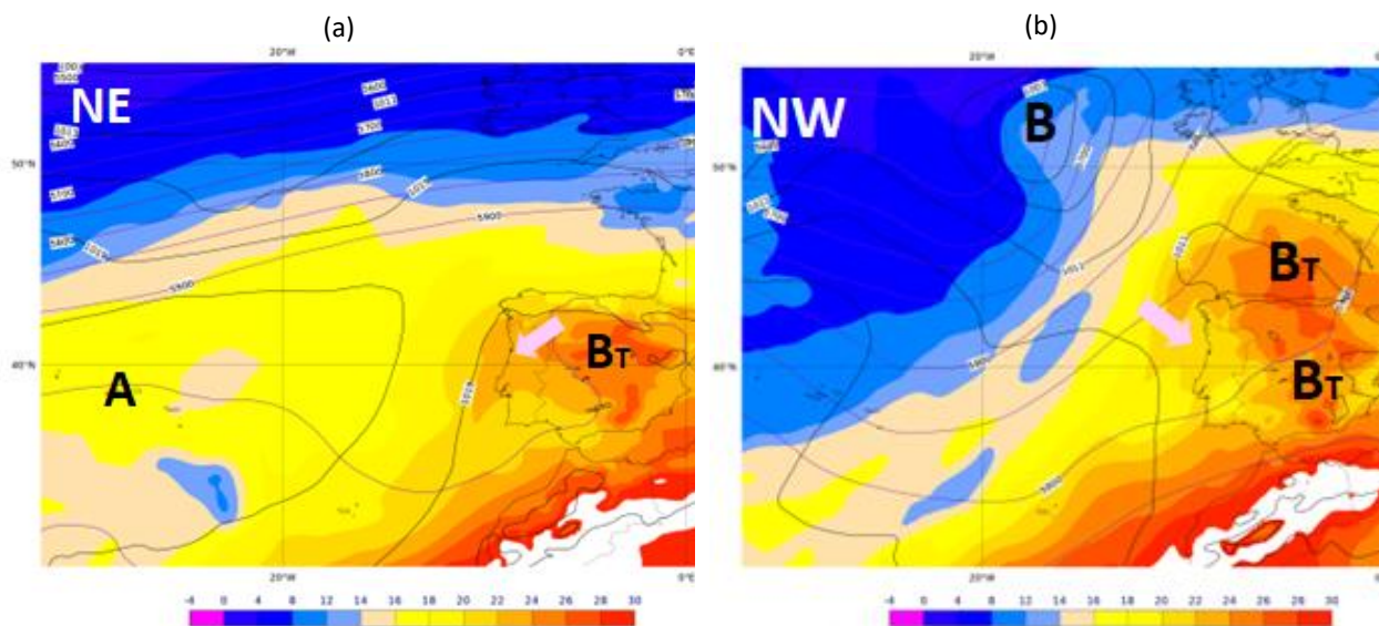
Figura 1 - Tipos de Tempo em agosto de 2024: ECMWF(ERA5) às 12 UTC. Pressão ao nível médio do mar às 12 UTC (linhas a preto, 4 em 4 hPa), altura do geopotencial aos 500 hPa (linhas violeta a tracejado, 50 em 50 m), temperatura aos 850 hPa (cor, °C). (a) WTNE (fluxo de nordeste, 9 agosto), (b) WTNW (fluxo noroeste, 11 agosto). - Anticiclone, B- Depressão, B T - Depressão Térmica, seta a violeta - direção do fluxo.
