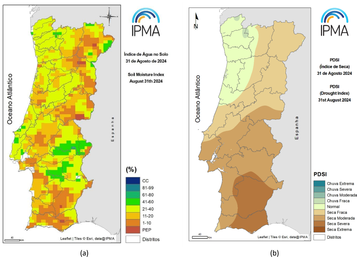
Figura 4 - Distribuição espacial em 31 de agosto de 2024 do teor de Água no Solo e da Seca, (a) percentagem de água no solo (média 0-100 cm profundidade), em relação à capacidade de água utilizável pelas plantas (ECMWF), (b) índice de seca, PDSI.
