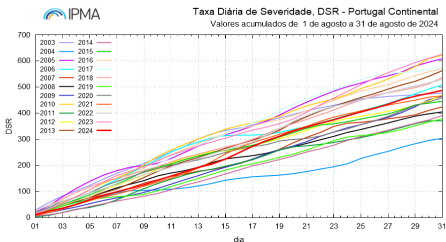
Figura 8 (b) - Evolução dos valores acumulados da taxa diária de severidade, DSR, no mês de agosto nos anos de 2003 a 2024.
