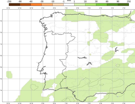
ECMWF - Anomalia Semanal da precipitação total Previsão de 20250326, válida para semana de 20250414 00H00 a 20250421 00h00
