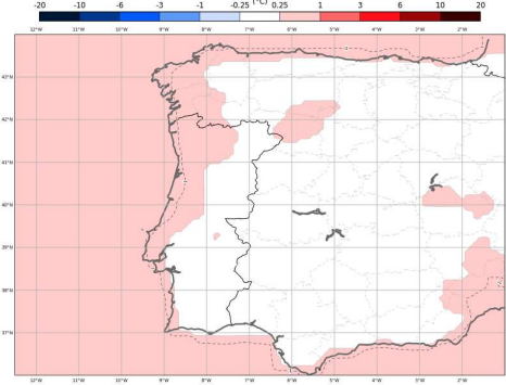
ECMWF - Anomalia Semanal da Temperatura a 2 metros Previsão de 20250326, válida para semana de 20250414 00H00 a 20250421 00h00
