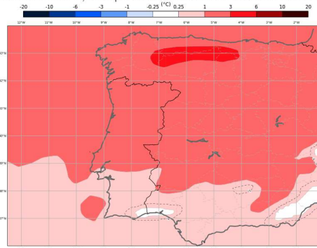
ECMWF - Anomalia Semanal da Temperatura a 2 metros Previsão de 20250326, válida para semana de 20250331 00H00 a 20250407 00h00
