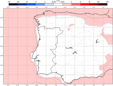
ECMWF - Anomalia Semanal da Temperatura a 2 metros Previsão de 20250326, válida para semana de 20250421 00H00 a 20250428 00h00
