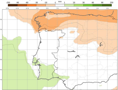
ECMWF - Anomalia Semanal da precipitação total Previsão de 20250326, válida para semana de 20250331 00H00 a 20250407 00h00
