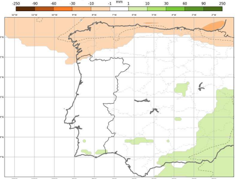
ECMWF - Anomalia Semanal da precipitação total Previsão de 20250326, válida para semana de 20250407 00H00 a 20250414 00h00
