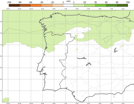
ECMWF - Anomalia Semanal da precipitação total Previsão de 20250326, válida para semana de 20250421 00H00 a 20250428 00h00
