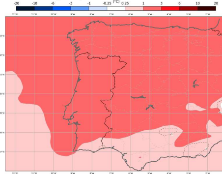
ECMWF - Anomalia Semanal da Temperatura a 2 metros Previsão de 20250326, válida para semana de 20250407 00H00 a 20250414 00h00
